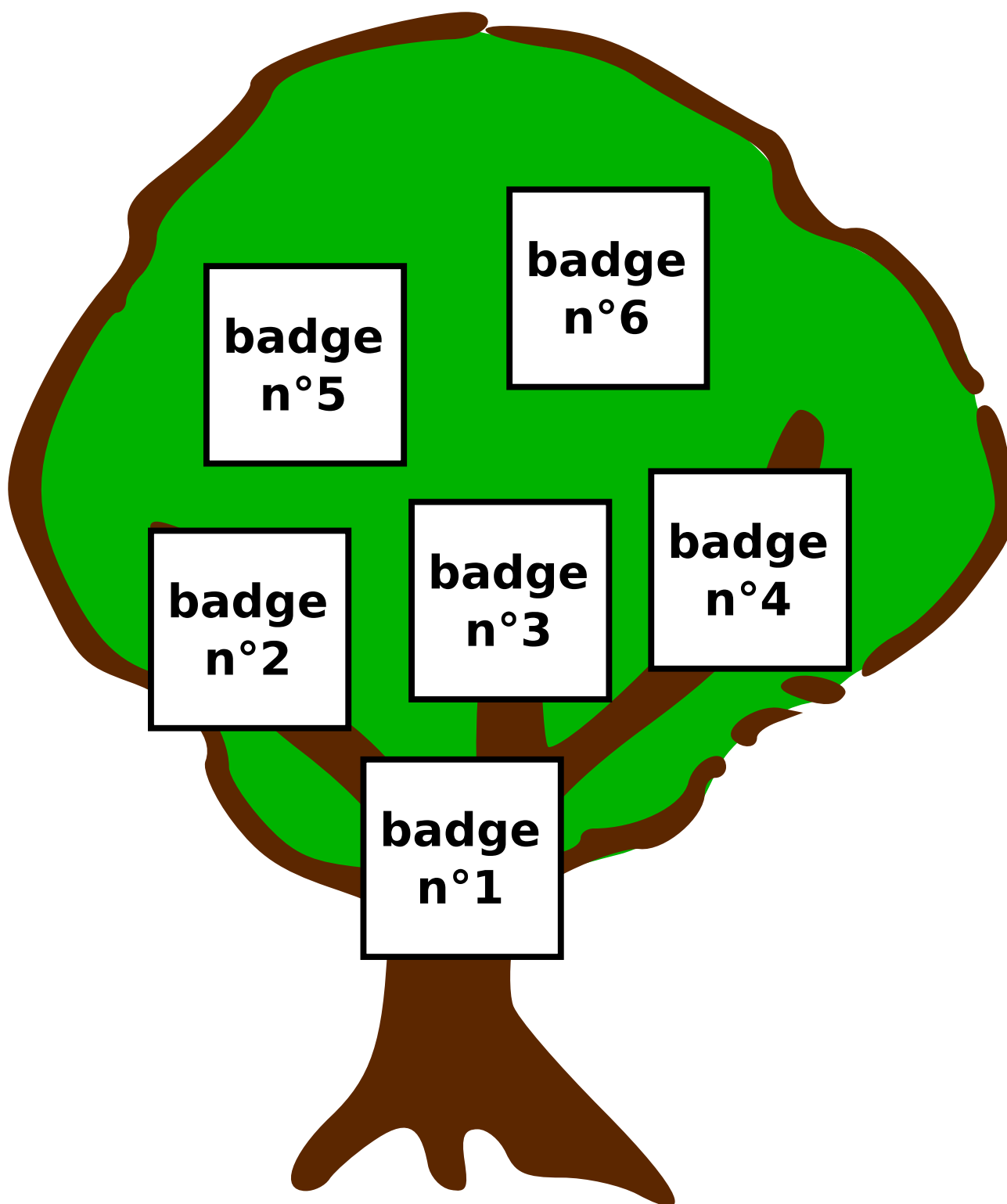
Arbre 14 : Sécher
